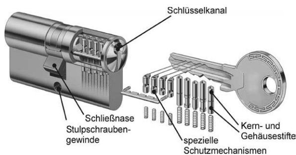
Bild 3-16: Aufbau eines Profilzylinders
