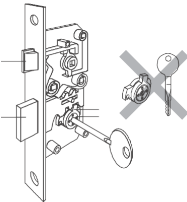
Bild 3-15: Zylindereinbausicherung
