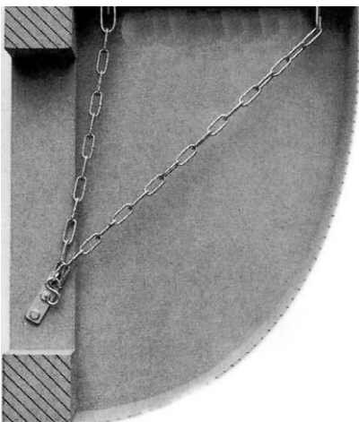
Bild 3-49: Befestigung im Mauerwerk beim Kunststofflichtschacht
