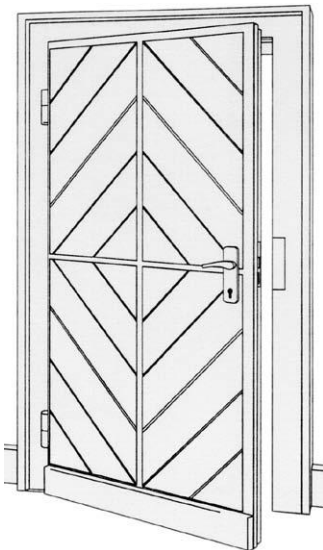
Bild 3-4: Vollholztür
