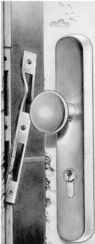
Bild 3-23: Ausgerissenes Schließblech
