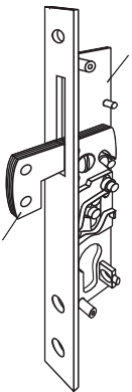
Bild 3-12: Haken-Schwenkriegelschloss
