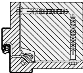
Bild 3-7: Eckzarge
