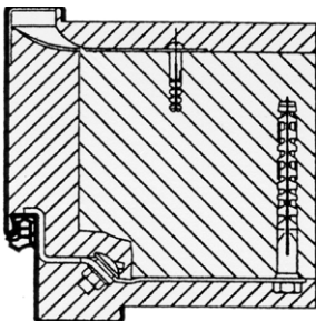
Bild 3-6: Mauerumfassende Stahlzarge
