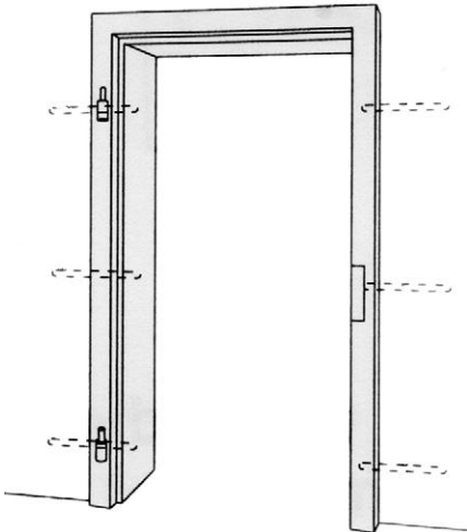
Bild 3-5: Türzarge
