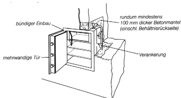
Bild 4-3: Einmauerschrank
