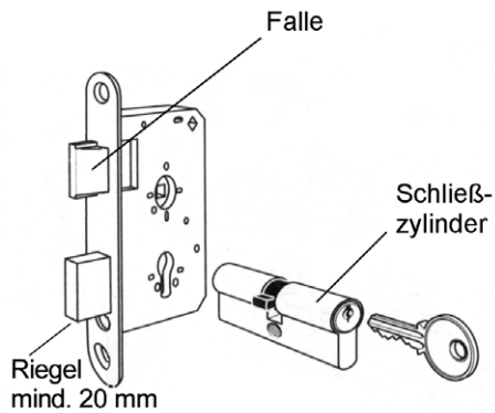
Bild 3-8: Zylindereinsteckschloss
