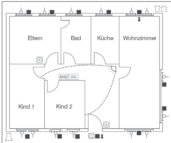
Bild 5-2: Außenhautüberwachung 1)
