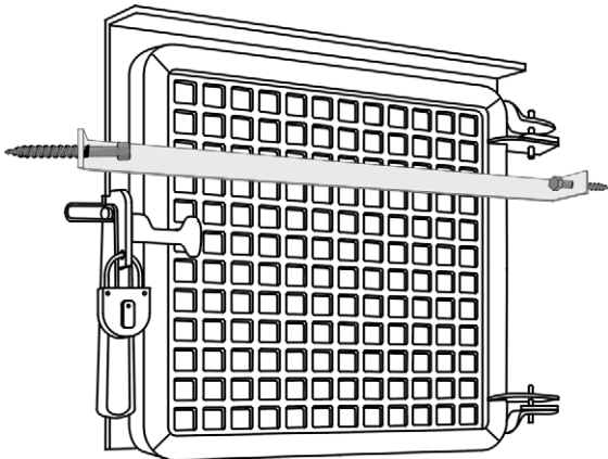
Bild 3-46: Gesicherte Stahllochblende
