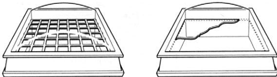
Bild 3-52: Lichtkuppel mit Gitter oder zusätzlicher einbruchhemmender Verglasung
