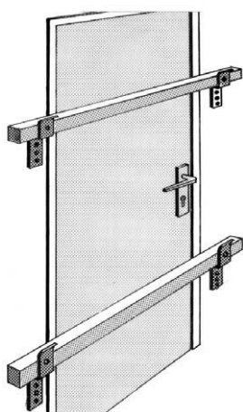
Bild 3-30: Tür mit Vorlegestangen
