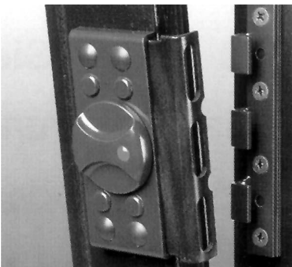
Bild 3-40: Bandseitensicherung
