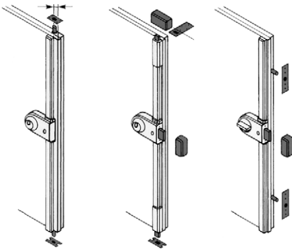
Bild 3-10: Aufsatzschlösser mit Mehrpunktverriegelung
