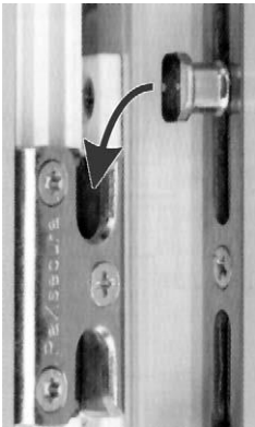
Bild 3-36: Pilzkopf mit Gegenstück
