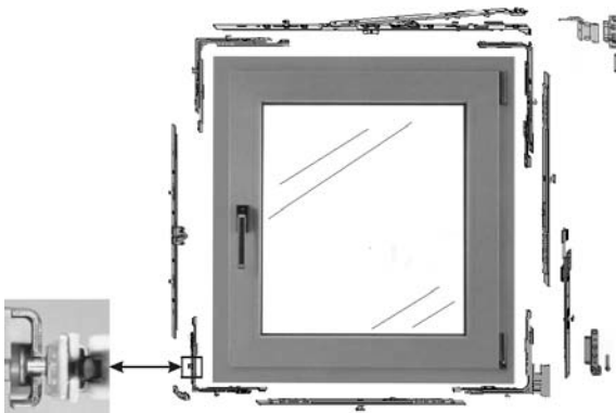
Bild 3-34: Einbruchhemmender Fensterbeschlag
