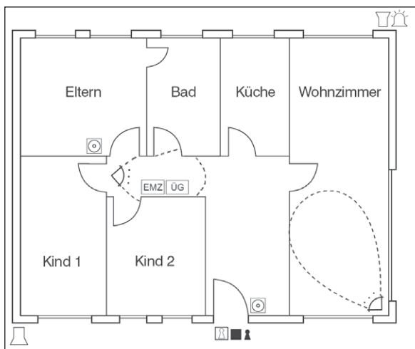
Bild 5-3: Schwerpunktüberwachung 1)
