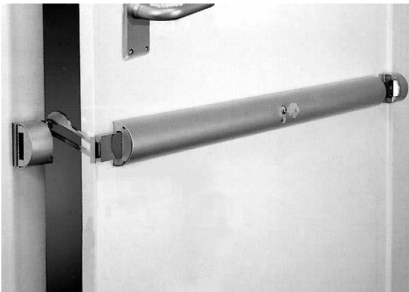
Bild 3-29: Querriegelschloss mit Sperrbügel
