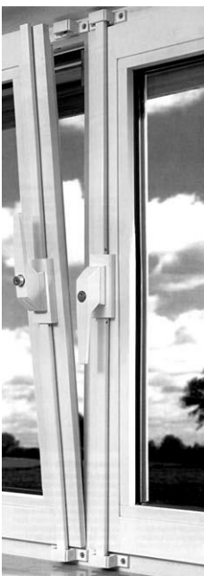
Bild 3-43: Fensterstangenschloss
